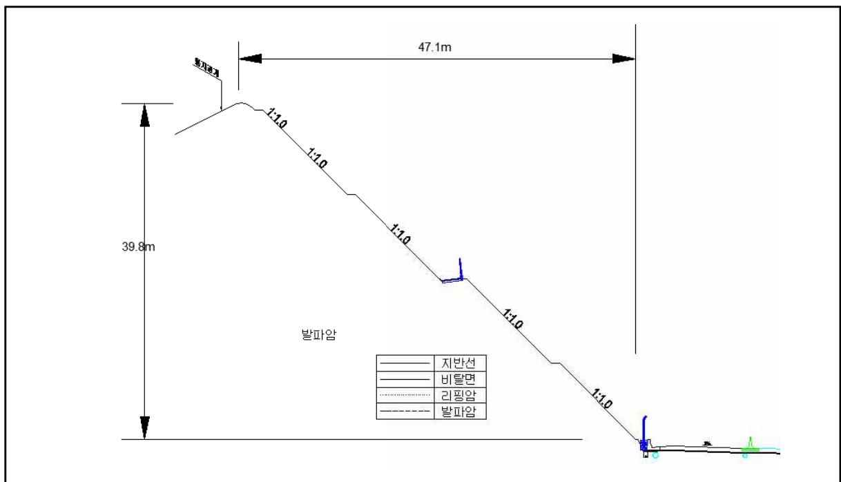
【대표단면 Sta.5+060(영천)】
