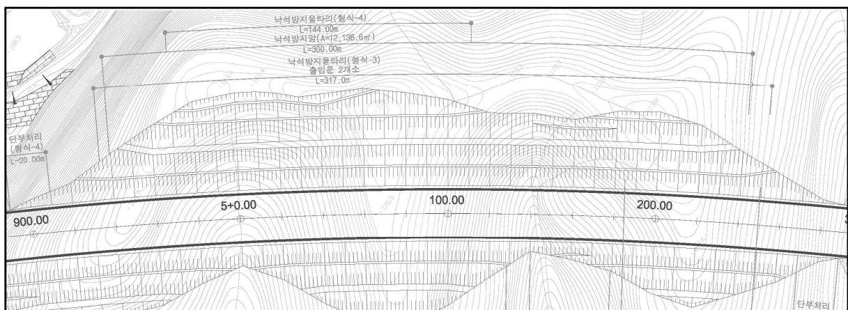
【Sta.4+900~5+300】
