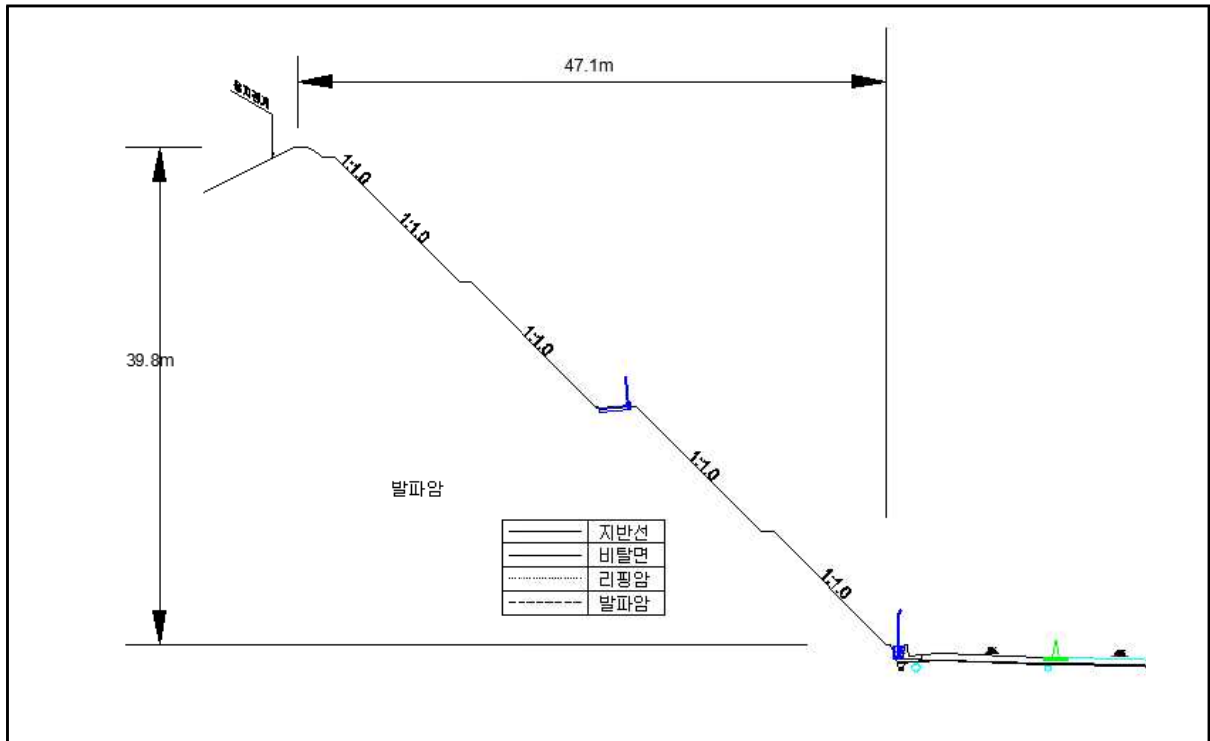
【대표단면 Sta.5+060(영천)】
