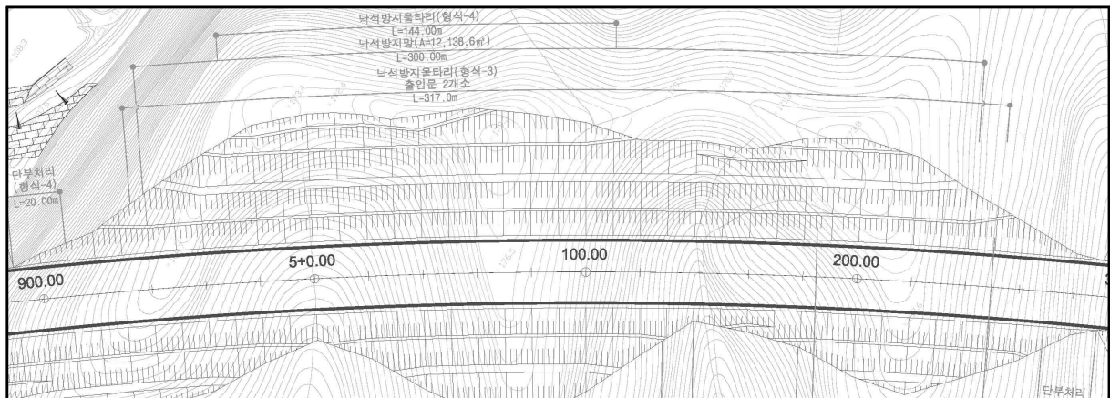
【Sta.4+900~5+300 평면】
